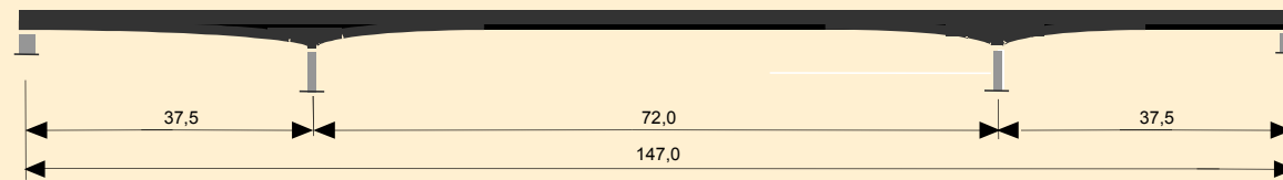
Oldalnézet
