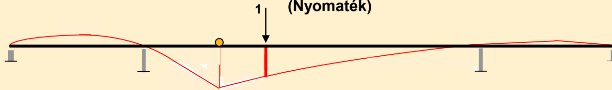
Kereszteloszlási ábra (Minden igénybevételre azonos)
